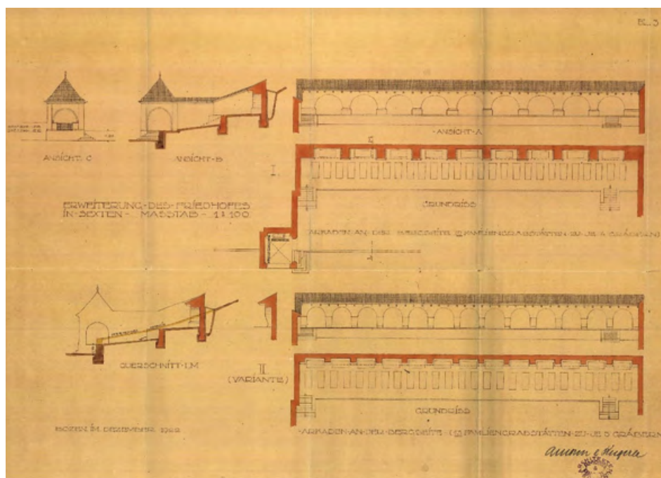
8.1 / 8.2 Marius Amonn & August Fingerle, Wettbewerbsentwurf Erweiterung des Friedhofes in Sexten, 1922. Aus: Bauarchiv der Gemeinde Sexten. © GA Sexten. Abbildung mit Genehmigung.
