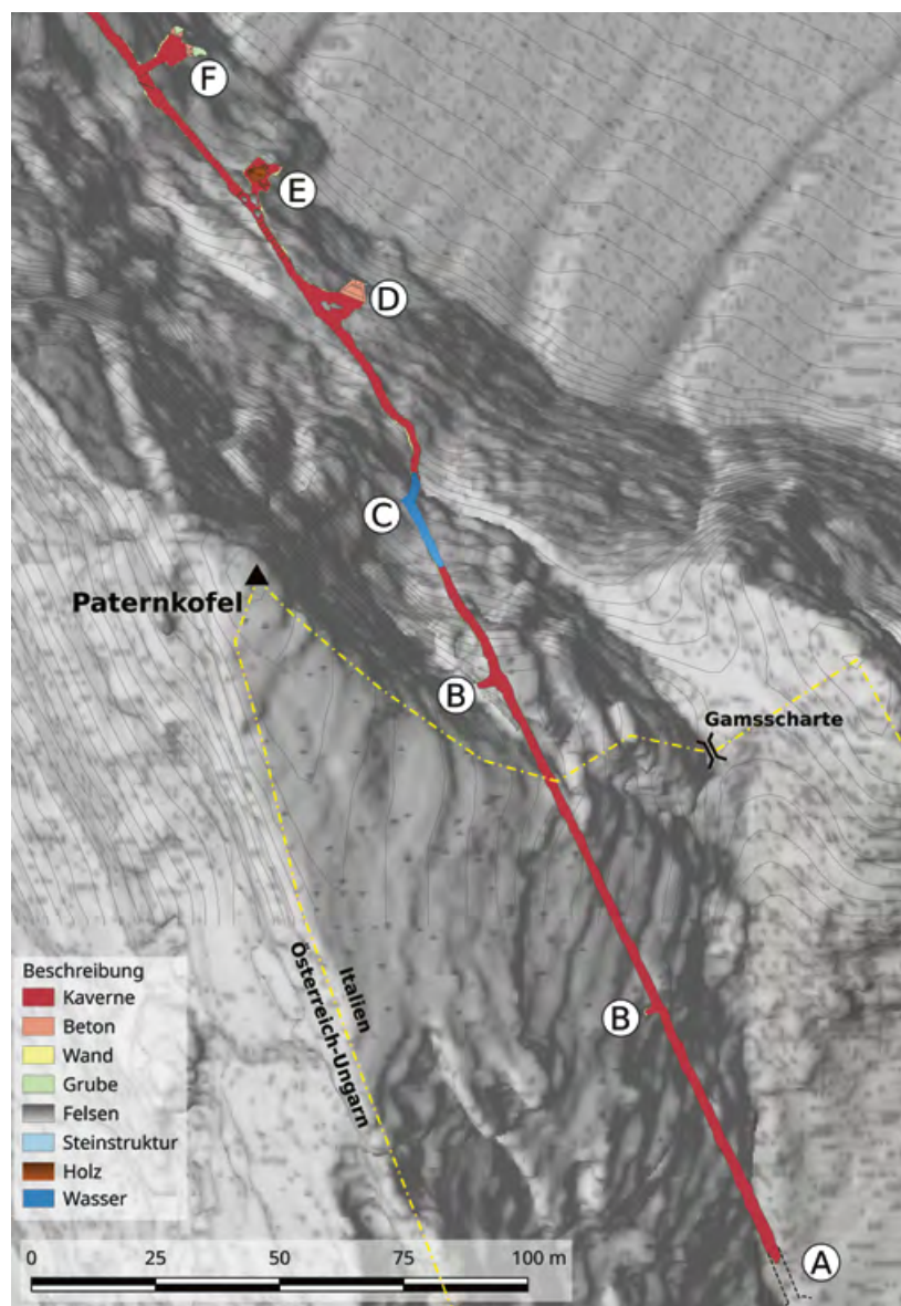
7 Bauabschnitt 1 des Paternkofelstollens. © 2021, unibz, WiL Archive. Abdruck mit Genehmigung.
