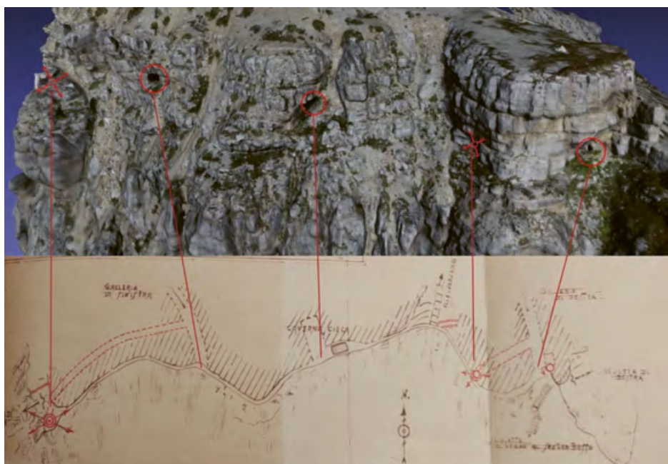
12 Sexten Alto. Andamento planimetrico della cengia collegante gli accessi alle gallerie, scala 1:400, estate 1917. Fonte: Archivio Ufficio Storico dello Stato Maggiore dell'Esercito, Roma, Carteggio 1917, I corpo d'armata, genio, sistemazione difensiva, B1110D 29A. © AUSSME. Riproduzione autorizzata. Confronto con ricostruzione 3D eseguita nel corso della campagna di rilievo del progetto "Written in the Landscape" nell'estate 2021, su cui sono stati evidenziati gli ingressi alle gallerie e le postazioni per mitragliatrice. © 2021, unibz, WiL Archive. Riproduzione autorizzata.
